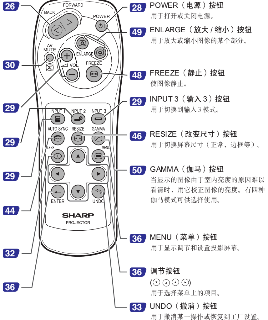
遥控信号发射器
